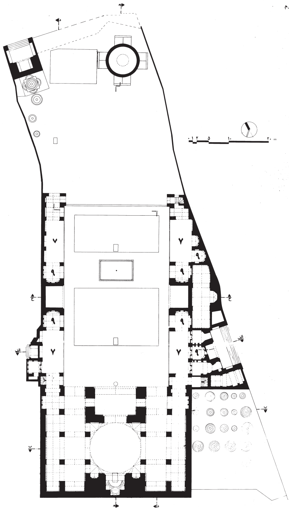
نقشه ۲. پلان طبقه دوم مسجد - مدرسه رحیم خان اصفهان (مأخذ: حاج قاسمی، ۱۳۷۵).
