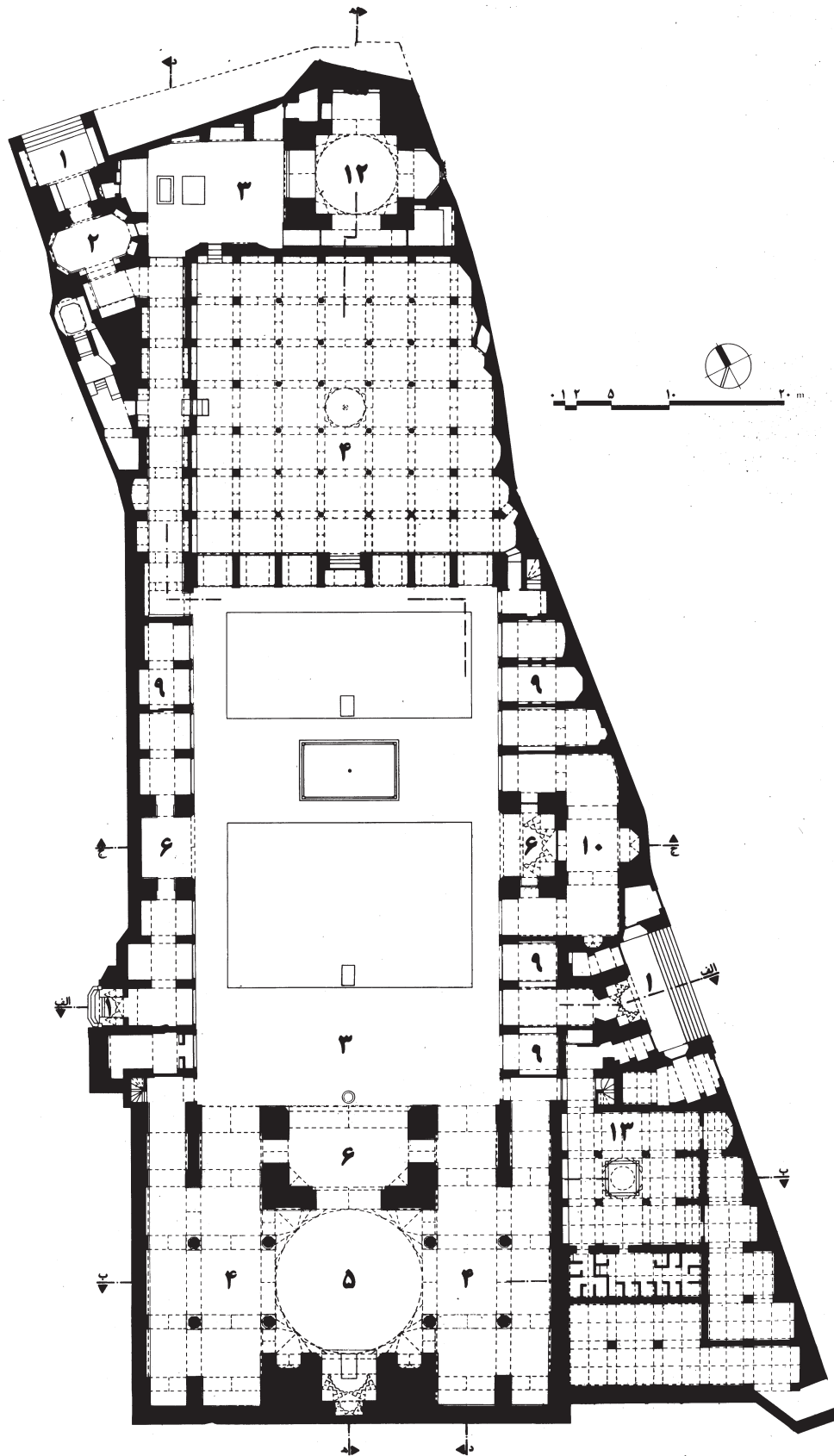
نقشه ۱. پلان طبقه اول مسجد - مدرسه رحیم خان اصفهان (مأخذ: حاج قاسمی، ۱۳۷۵).
